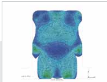
有限元分析 (FEA) 通过二维分析可实现气缸盖罩密封垫与密封垫沟槽的优化对准。
